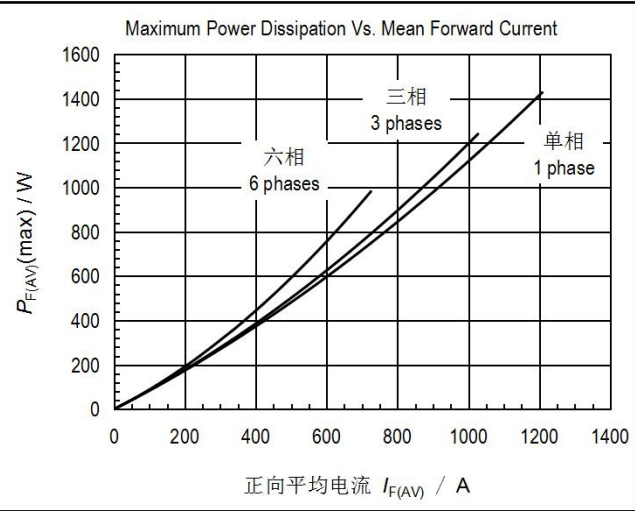
图3. 最大正向功耗与正向平均电流的关系曲线
